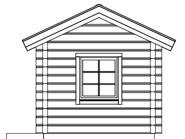
FASAD MOT HÖGER
