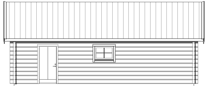
FASAD MOT VÄNSTER
